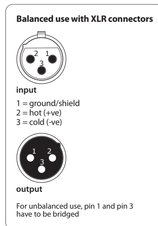
Fig. 8.1: Connecteur XLR
