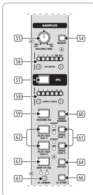
Fig. 5.1: La section sampleur
