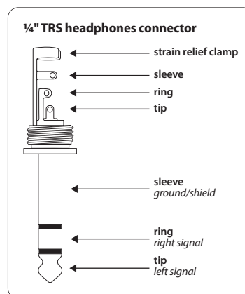
Fig. 8.2: Sortie casque sur jack stéréo
