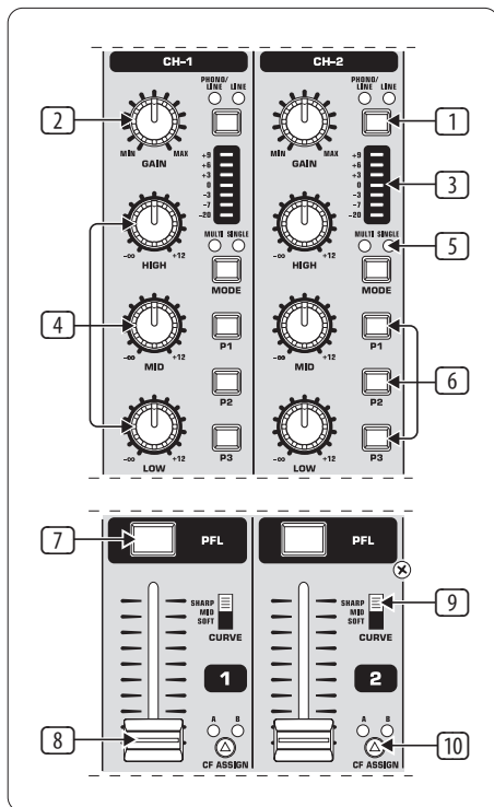
Fig. 2.1: Les canaux stéréo
