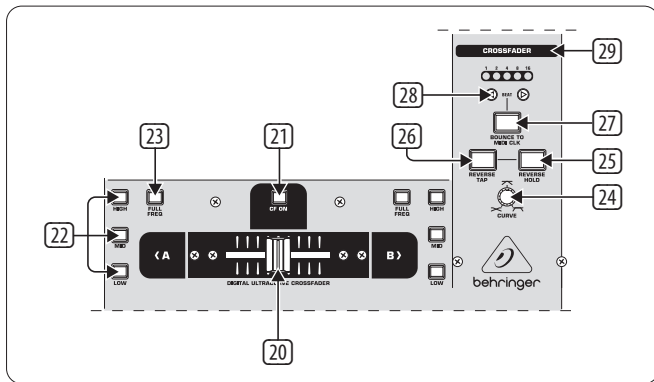
Fig. 2.3: La section crossfader
