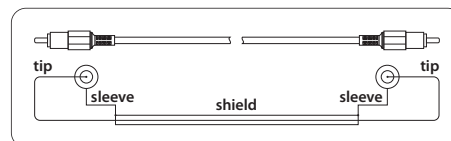
Fig. 8.3: Câble RCA
