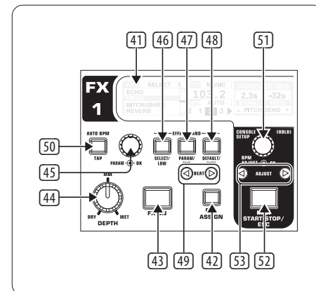
Fig. 4.2: La section d'effets (ici: FX 1)
