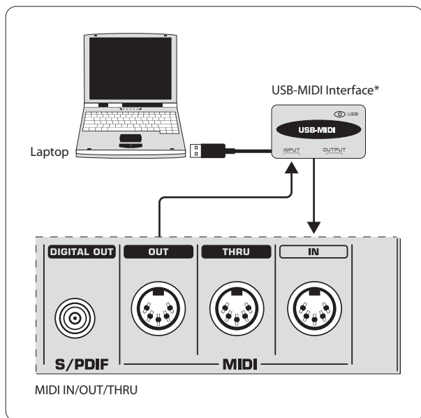
Fig. 7.1: Raccordement de la DDM4000 à un ordinateur
