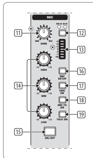
Fig. 2.2: Le canal micro
